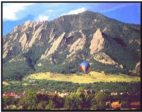
input
